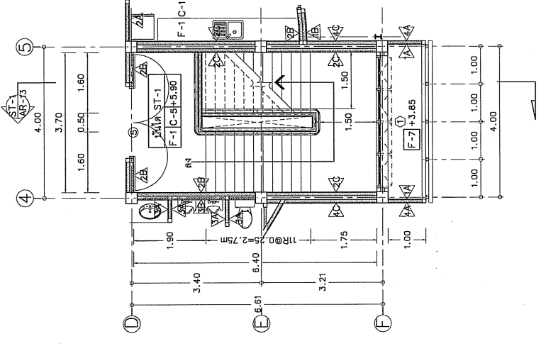
แปลนขยายบันไดชุด 1 ST-1 ขนาดเท่าจริง
